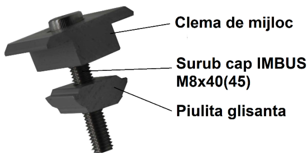
Fig. 1 Clema fixare de mijloc – Parti componente
