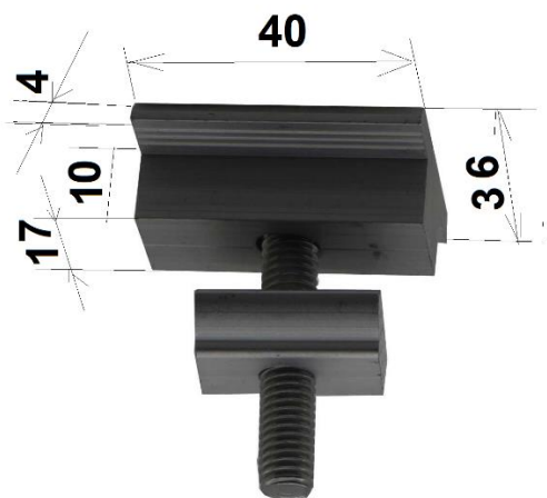
Fig. 2 Dimensiuni clema de mijloc
