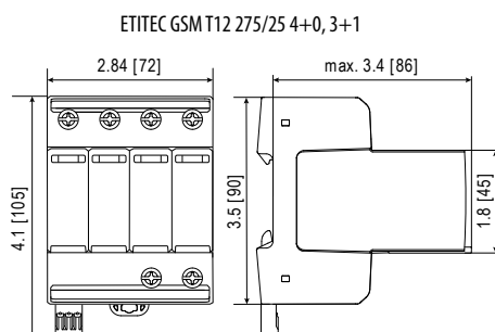
MOD. ETITEC GSM T12 275/25
