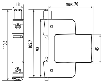
ETITEC ML T123 300/12,5 (1+0) RC
