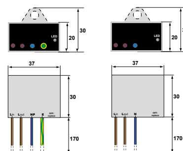
ETITEC LX1 IP67
